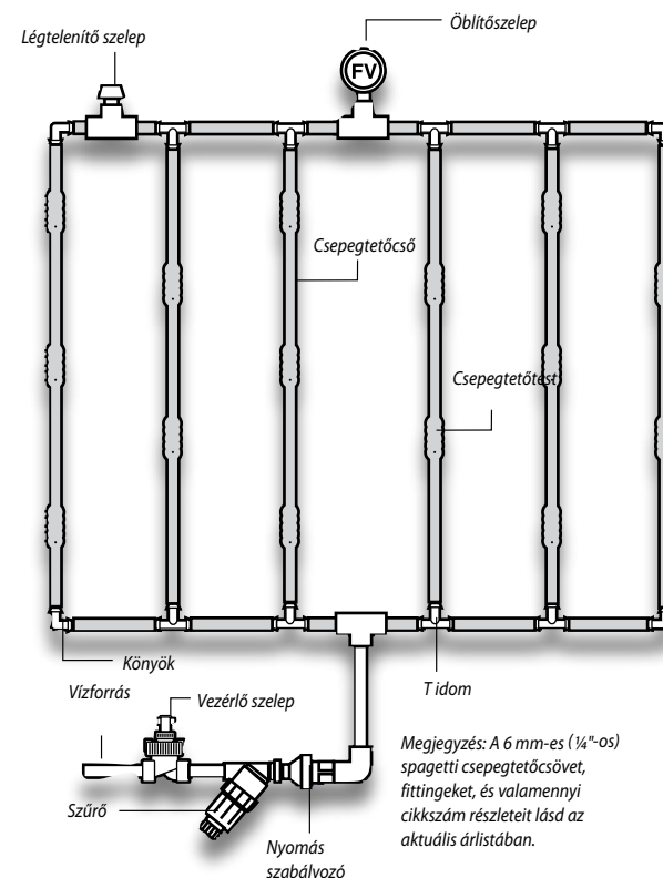
Tipikus felszín alatti csepegtető öntözőrendszer terve
