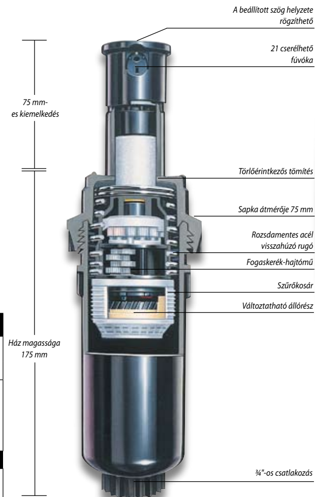
Super 700-as gyepöntöző, kiemelkedő
