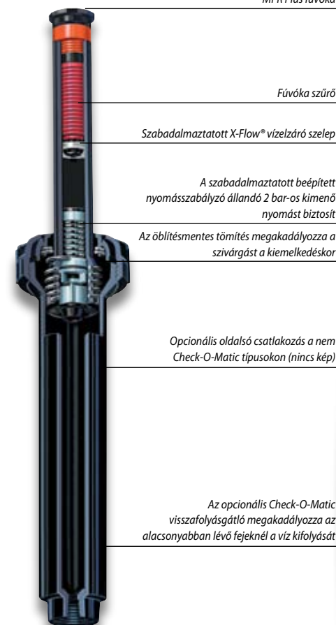
570Z PRX sorozat
